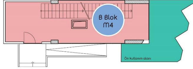
ZEMİN KAT PLANI - MAĞAZA
